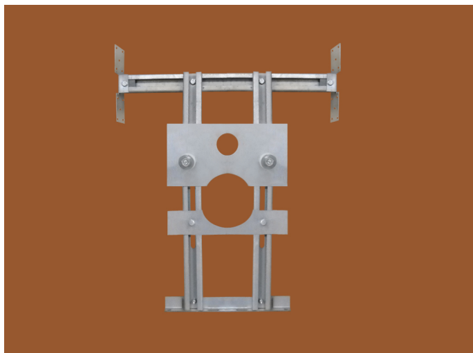
ART.83/R:TELAIO PER WC SOSPESO SU PARETI IN CARTONGESSO
