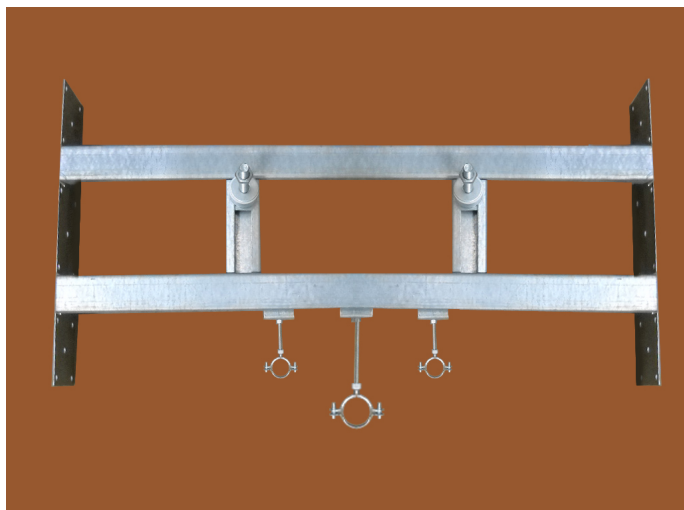
ART.83/H:TELAIO REGOLABILE PER LAVABO SU PARETI IN CARTONGESSO
