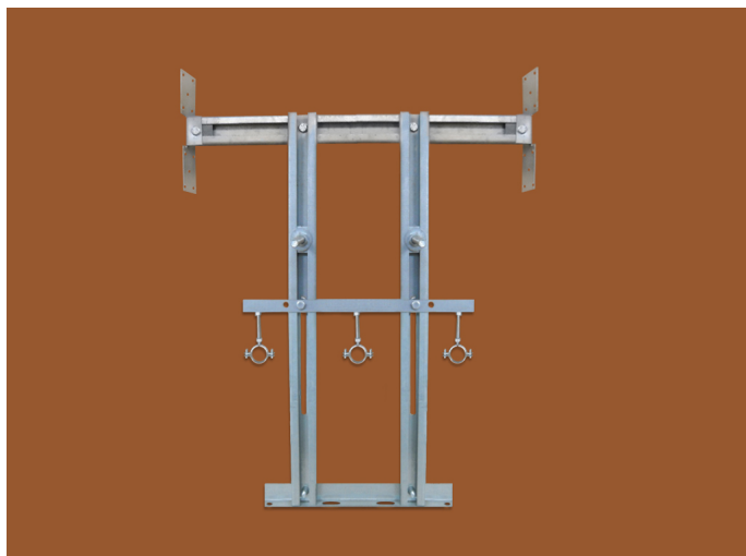
ART.83/O:TELAIO PER BIDET SOSPESO SU PARETI IN CARTONGESSO
